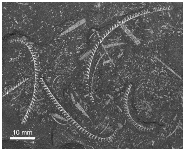
Vyhybný prvohorní živočich – graptolit Demirastrites triangulatus
