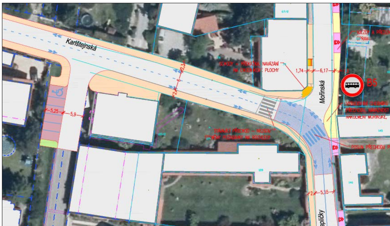
Obr. 2: Křižovatka u České hospody – navržen je posun přechodu tak, aby se chodci jdoucí na Mořinskou vyhnuli schodům před restaurací. Zároveň je navržen zákaz vjezdu pro autobusy směrem na Mořinu.
