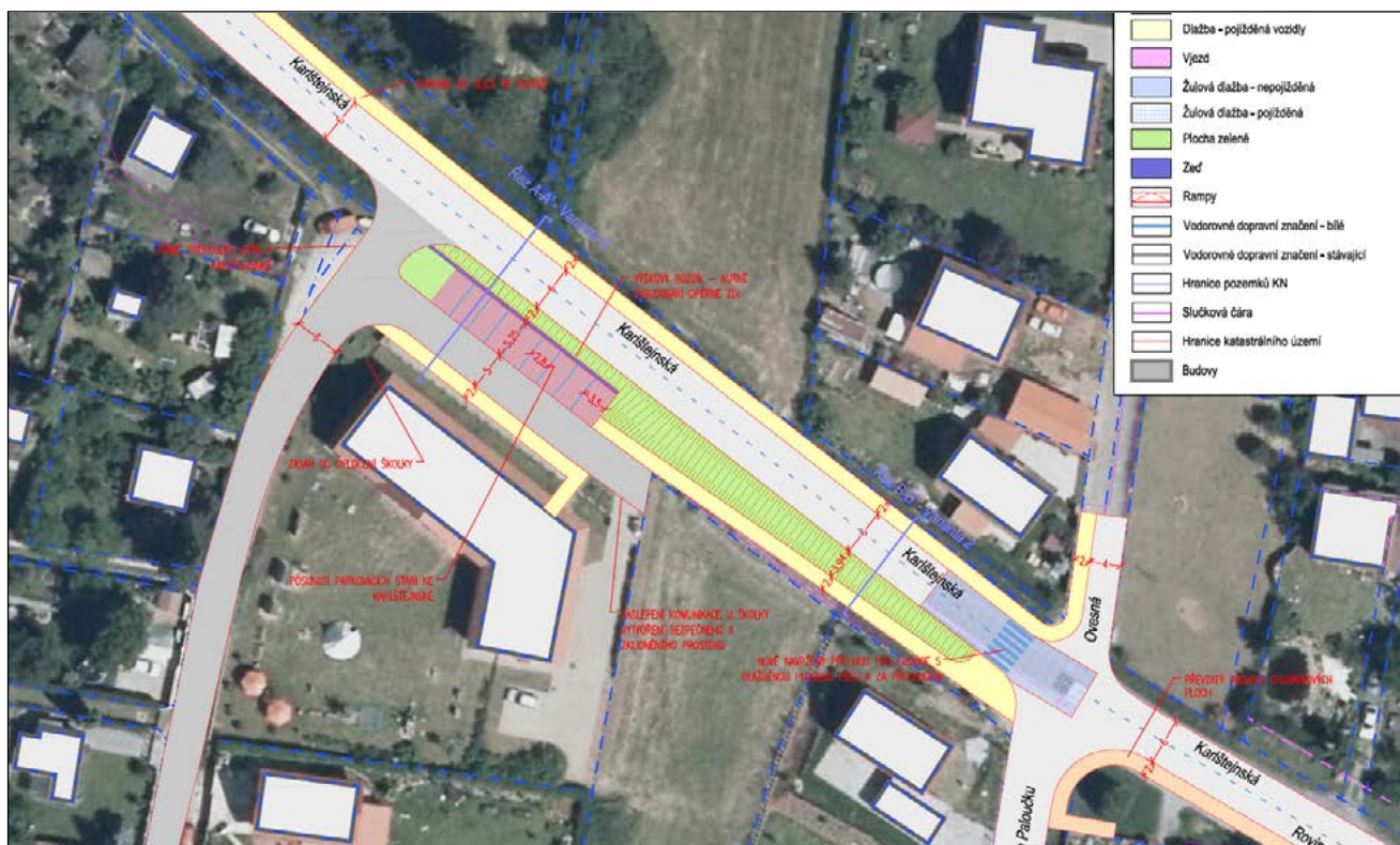
Obr. 4: Napojení ulice Luční na Karlštejskou – stávající část ulice od školky směrem ke křižovatce Na Paloučku je v návrhu nahrazena přímým napojením s úpravou prostoru před školkou. V návrhu je patrný také chodník na severní straně Karlštejské ulice.
