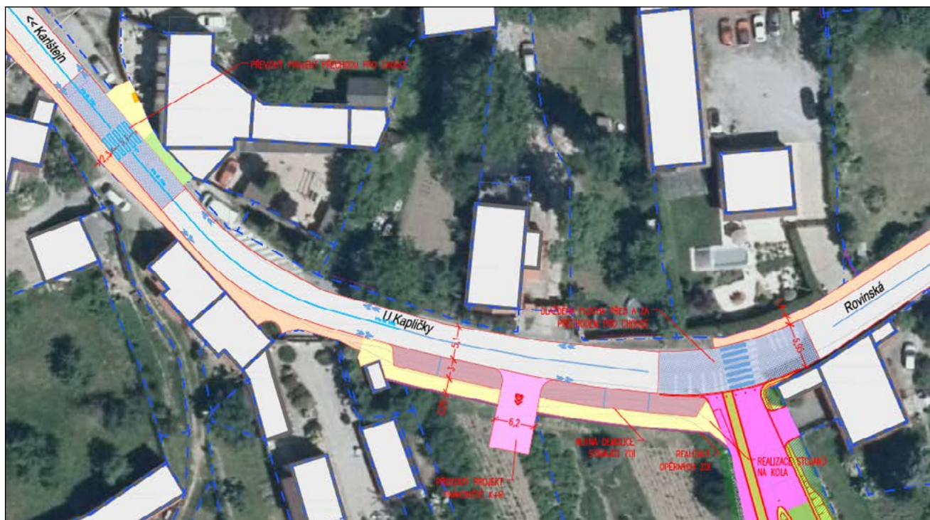
Obr. 3: Předprostor lávky – návrh pěti míst pro krátkodobé zastavení (parkoviště K+R) a změna povrchu vozovky v místech přechodů. Nově je navržen přechod na návsi u školy Hlásek.
