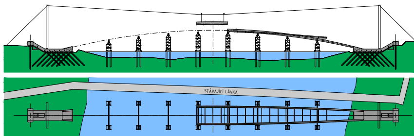
Montáž krajních polí mostovky
