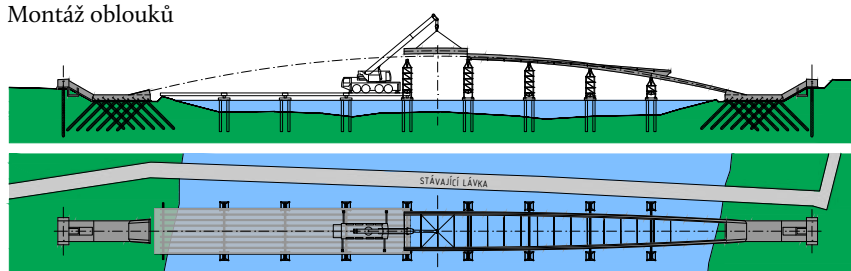
Montáž oblouků
