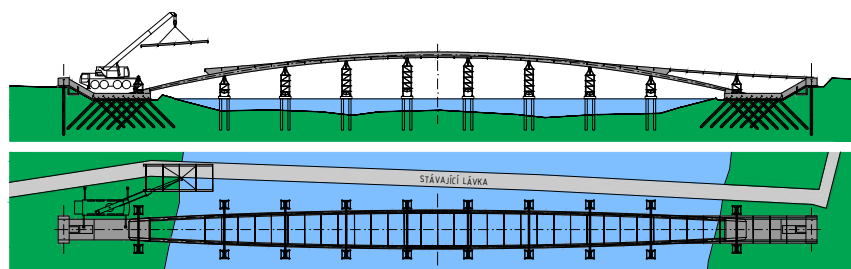
Montáž krajních polí mostovky
