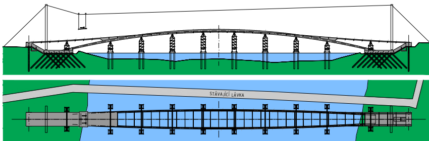
Pokládka betonových segmentů
