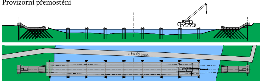
Provizorní přemostění
